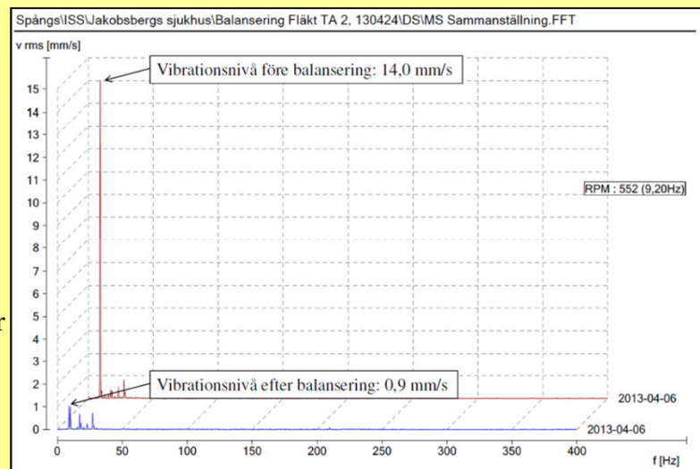
Resultat av balanseringen i form av minskade vibrationer.
