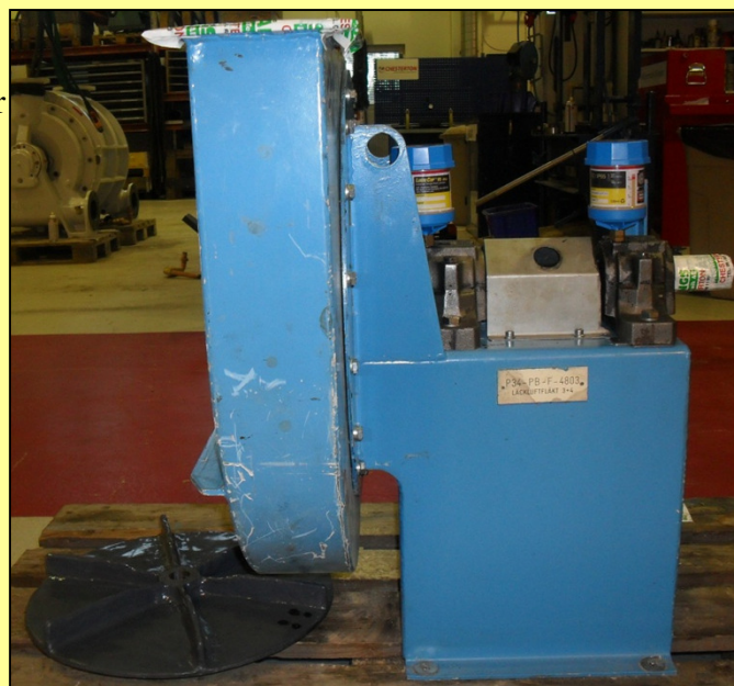
Kompositbelagd fläkt som används för transport av överblivet träpulver som härstammar från mald pellets.
