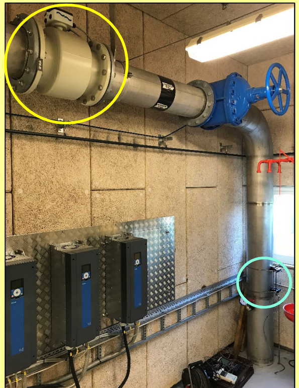
En av de två fasta flödesmätare (gul ring) som kontrollerades med vår mobila flödesmätare (turkos ring) på Nynäshamns reningsverk.
